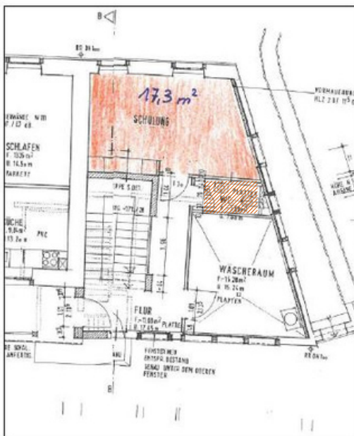
Erdgeschoss
